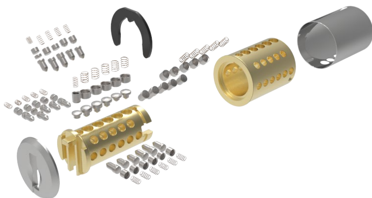
Bild 2 (Explosion Systemkapsel): Maximale Präzision: Die radiale Anordnung der Stiftzuhaltungen im Inneren des SEA-4.0m Schliesszylinders.
